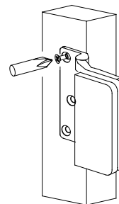
Obrázek 9: Připevníte závěs skleněných dveří.
