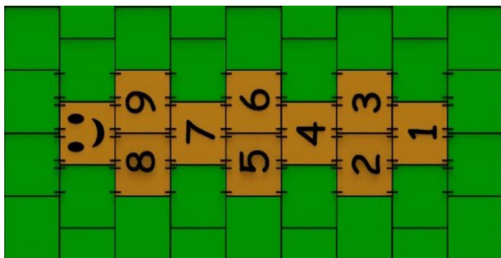
Obr.K5: Správná montáž dlaždic „skákací panák“
