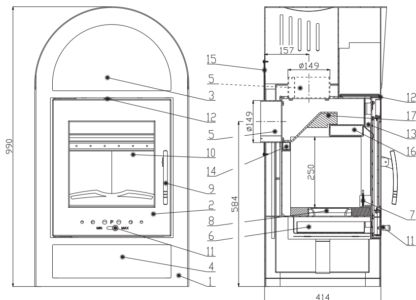
Šamotová vyzdívka
