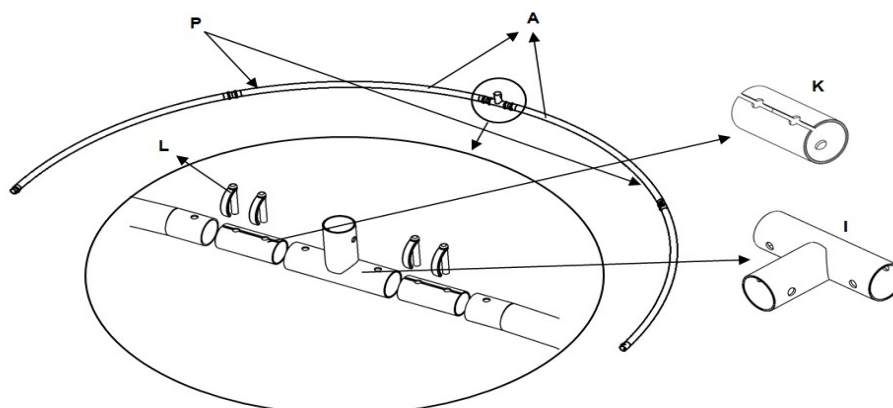
A Oblouk 40 mm (sestavené do polooblouku) I Držák jednostranný K Spojka L Kolík P popruhy oblouků Obrázek 2
