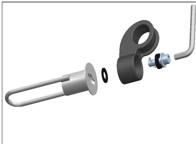
Obrázek G – sestava kotvy (zleva doprava):
