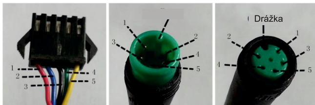
Zapojení displeje
